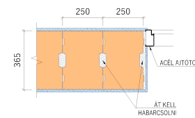
- KÖTÉS AZ AJTÓFALAZATNÁL, AZ 1. SOR FALAZAT
