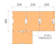
- SAROKKÖTÉS, A 2. SOR FALAZAT
