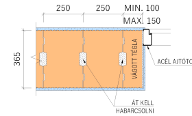
- KÖTÉS AZ AJTÓFALAZATNÁL, A 2. SOR FALAZAT
